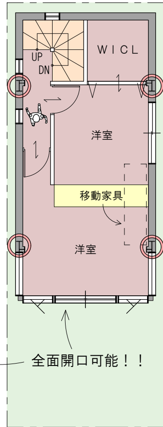
3 F 平面図
