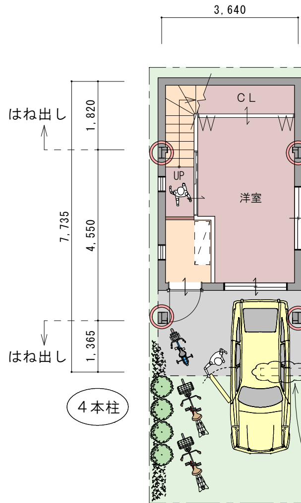
1 F 平面図
